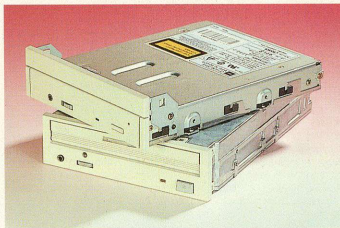
Toshiba XM-3401, XM-4101 B: High-End und Low-Cost, beides vom gleichen Hersteller. Eine gute Kombination.
